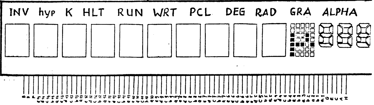
Fig.4 Display-Verdrahtung
